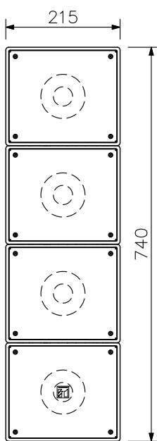
正面図
