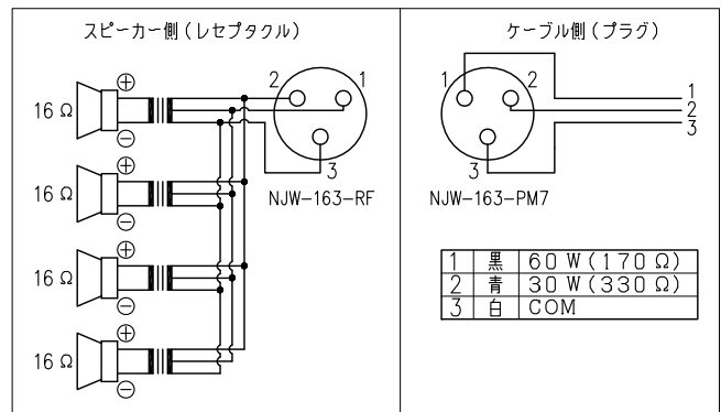
結線図
